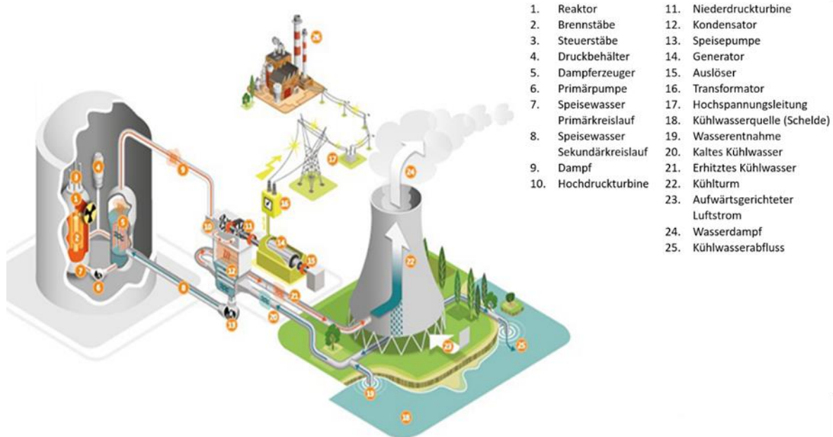
Abbildung 2: Betrieb eines Kernkraftwerks mit (von links nach rechts) dem Reaktorgebäude, dem Maschinenraum und dem Kühlkreislauf (Quelle: Electrabel AG).
